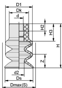
Конструктивные данные FG 12 HT1-60 N016
