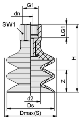
デザインデータ FSG 20 HT1-60 G1/8-IG
