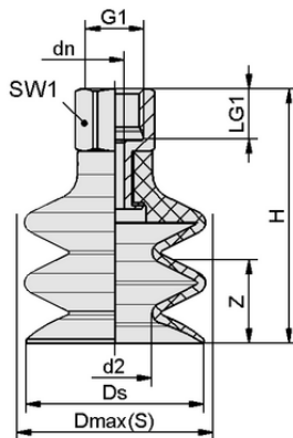
デザインデータ FSG 12 HT1-60 G1/8-IG
