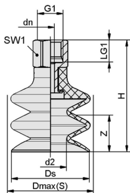
Dati di costruzione FSG 7 HT1-60 G1/8-IG
