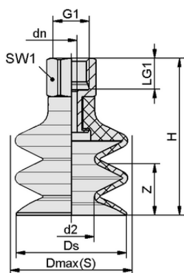
Données de construction FSG 7 HT1-60 G1/8-IG
