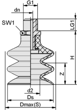
Tasarım verileri FSG 7 HT1-60 G1/8-AG
