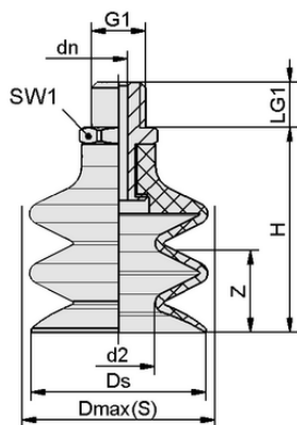
Конструктивные данные FSG 7 HT1-60 G1/8-AG
