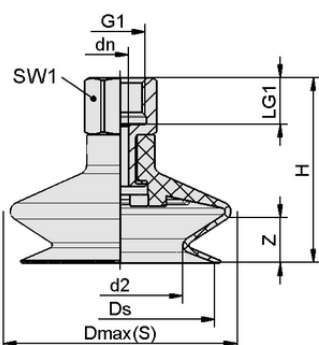
Datos de diseño FSGA 11 HT1-60 G1/8-IG
