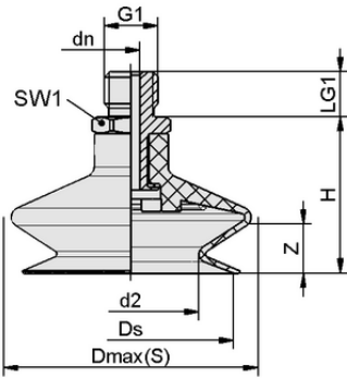
Tasarım verileri FSGA 16 HT1-60 M5-AG
