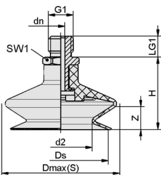
Конструктивные данные FSGA 16 HT1-60 M5-AG
