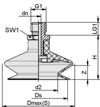
デザインデータ FSGA 11 HT1-60 G1/8-AG
