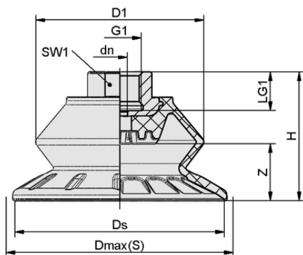
Конструктивные данные SAB 30 NBR-60 G1/4-IG
