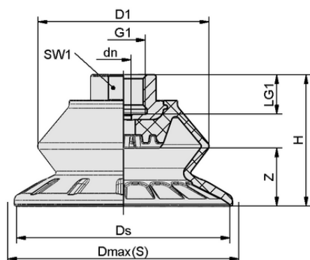
デザインデータ SAB 30 NBR-60 G1/4-IG
