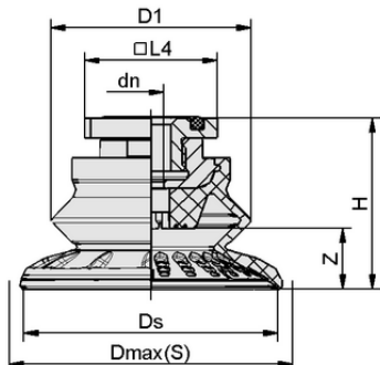
デザインデータ SAB 60 NBR-60 RA
