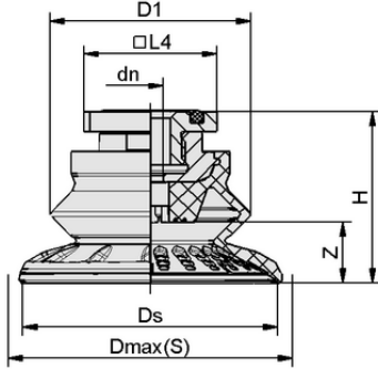
Tasarım verileri SAB 50 NBR-60 RA
