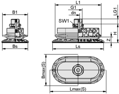
Tasarım verileri SAOB 140x70 NBR-60 M14x1.5-AG
