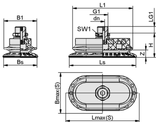
Datos de diseño SAOB 140x70 NBR-60 M10-AG
