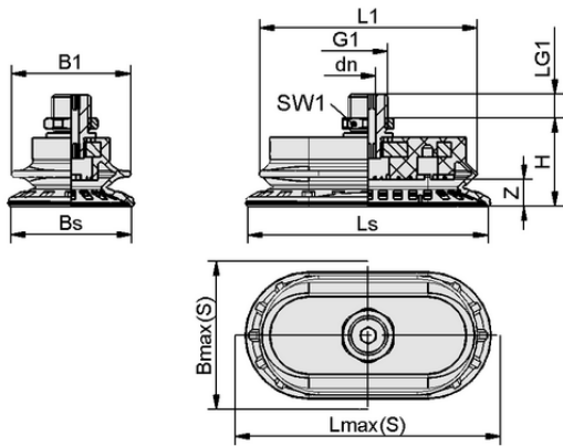
Données de construction SAOB 140x70 NBR-60 M10-AG
