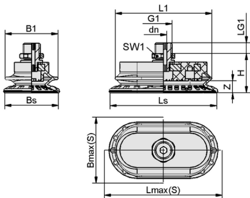
Données de construction SAOB 60x30 NBR-60 M10-AG
