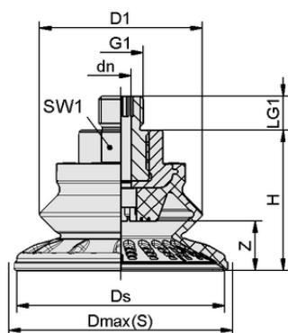
Конструктивные данные SAB 125 NBR-60 M14x1.5-AG
