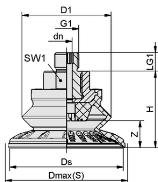
Конструктивные данные SAB 50 NBR-60 M14x1.5-AG
