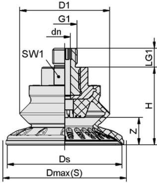
Tasarım verileri SAB 50 NBR-60 M14x1.5-AG
