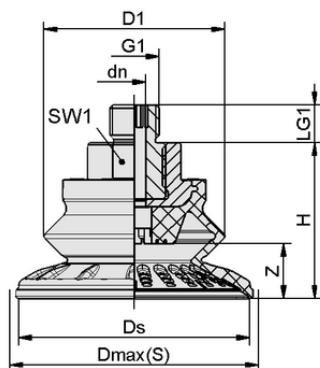
Конструктивные данные SAB 80 NBR-60 M10-AG
