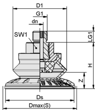
Конструктивные данные SAB 60 NBR-60 M10-AG
