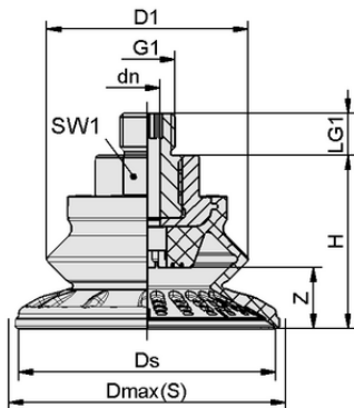
Datos de diseño SAB 40 NBR-60 M10-AG
