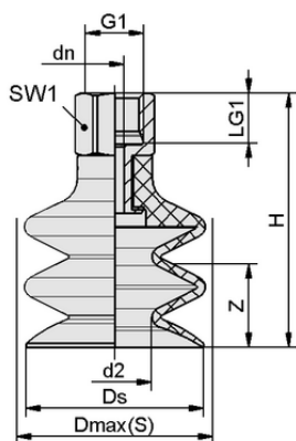
Datos de diseño FSG 25 HT1-60 G1/8-IG
