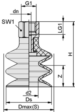
Tasarım verileri FSG 9 HT1-60 G1/8-IG
