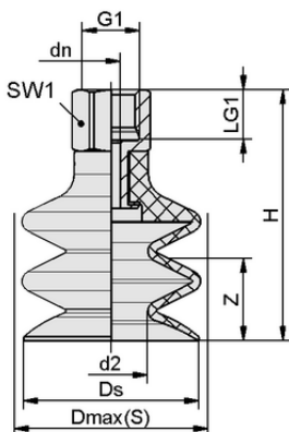
デザインデータ FSG 9 HT1-60 G1/8-IG
