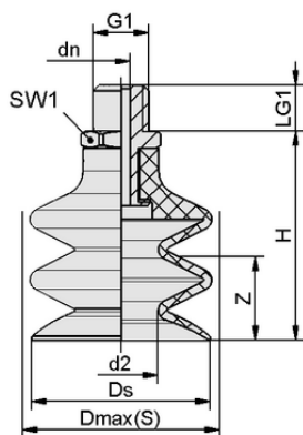
Dati di costruzione FSG 14 HT1-60 M5-AG
