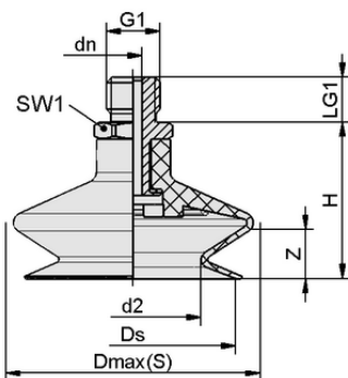
Dati di costruzione FSGA 14 HT1-60 M5-AG
