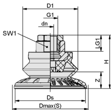
Конструктивные данные SAB 40 NBR-60 G3/8-IG
