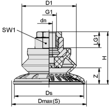
Tasarım verileri SAB 40 NBR-60 G3/8-IG
