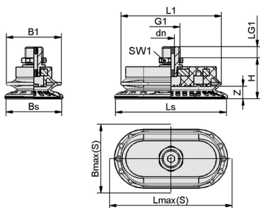
デザインデータ SAOB 110x55 NBR-60 G1/4-AG
