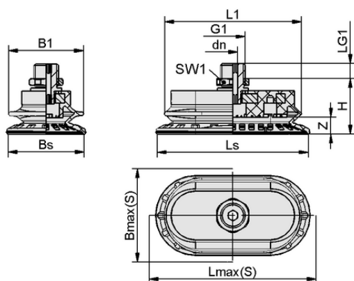
デザインデータ SAOB 80x40 NBR-60 G1/4-AG
