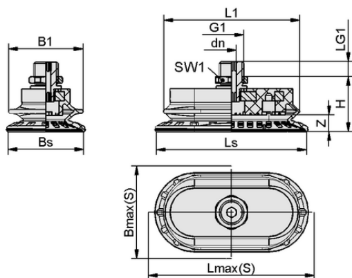
Datos de diseño SAOB 80x40 NBR-60 G1/4-AG
