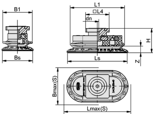
Données de construction SAOB 110x55 NBR-60 RA
