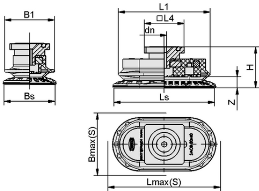
Design data SAOB 80x40 NBR-60 RA
