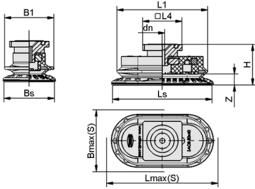
Tasarım verileri SAOB 80x40 NBR-60 RA
