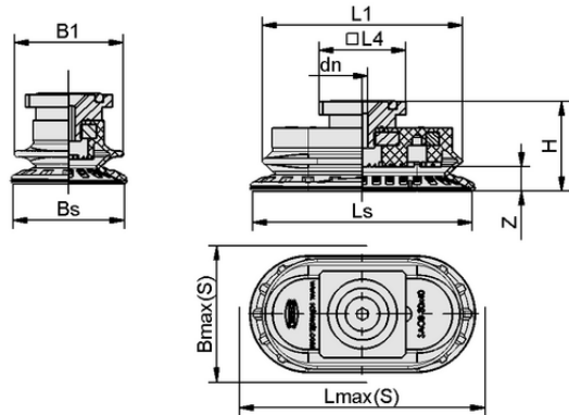
デザインデータ SAOB 60x30 NBR-60 RA
