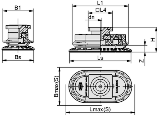
Tasarım verileri SAOB 60x30 NBR-60 RA
