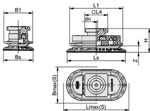
Конструктивные данные SAOB 60x30 NBR-60 RA
