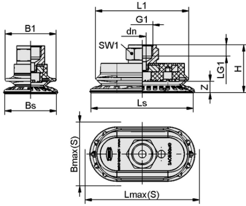
Tasarım verileri SAOB 80x40 NBR-60 G3/8-IG
