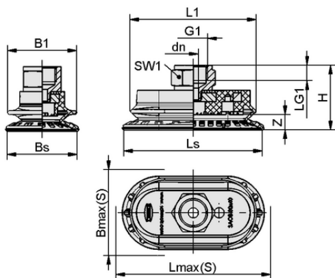
Datos de diseño SAOB 80x40 NBR-60 G3/8-IG
