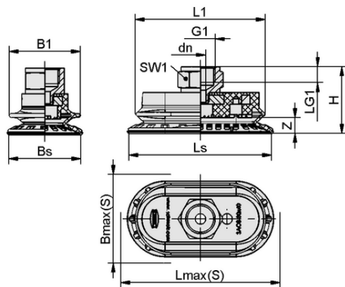
Конструктивные данные SAOB 80x40 NBR-60 G3/8-IG
