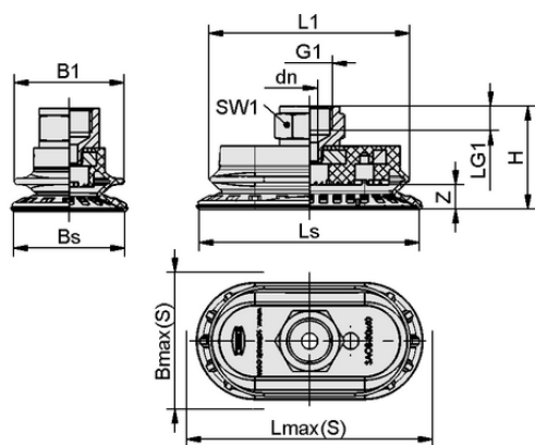
デザインデータ SAOB 110x55 NBR-60 G1/4-IG
