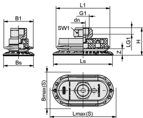
Données de construction SAOB 140x70 NBR-60 G3/8-IG
