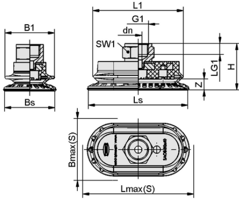
Tasarım verileri SAOB 110x55 NBR-60 G3/8-IG
