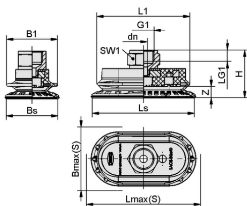
デザインデータ SAOB 110x55 NBR-60 G3/8-IG
