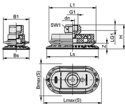
Конструктивные данные SAOB 60x30 NBR-60 G1/4-IG
