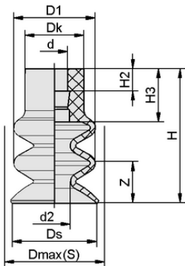
Datos de diseño FG 25 HT1-60 N016
